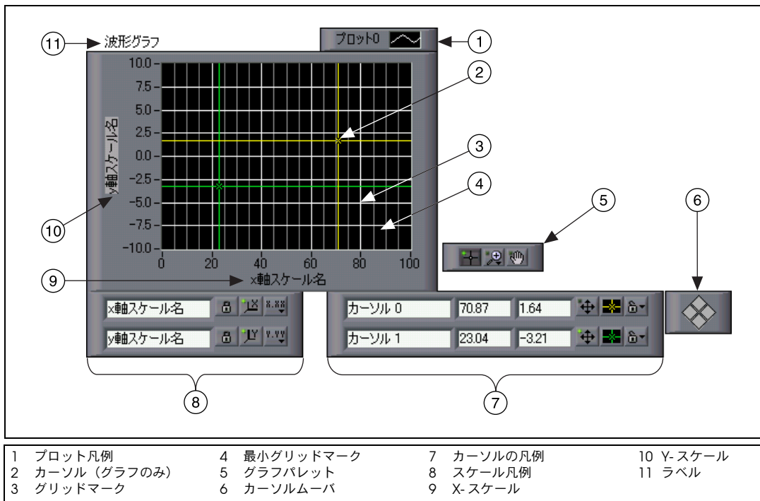
図 12-1 グラフの要素
