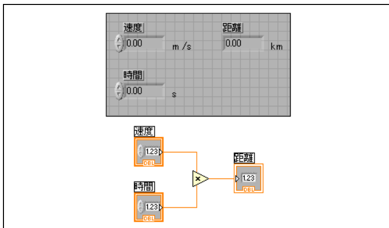
図 7-5 単位に互換性があるオブジェクトの配線
