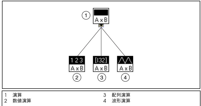
図 7-3 多態性 VI の例
