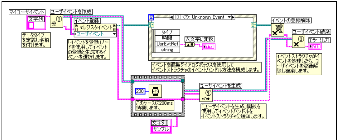
図 9-3 ユーザーイベントを生成する
