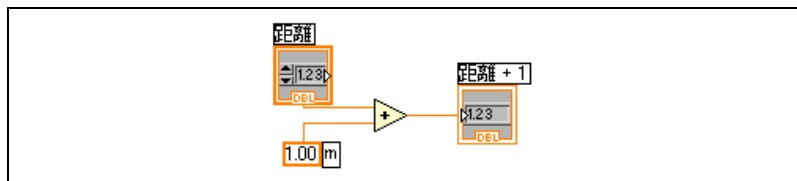
図 7-7 単位を持つ「インクリメント」関数の作成
