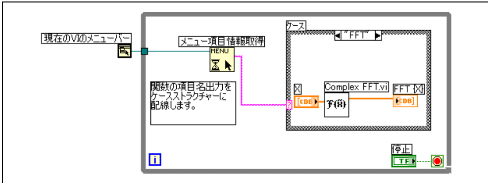
図 16-1 メニュー処理を使用したブロックダイアグラム
