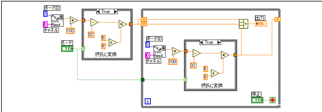
図 6-1 2つの同じ操作を持つブロックダイアグラム
