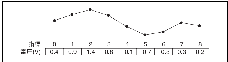
図 10-3 数値配列の波形
