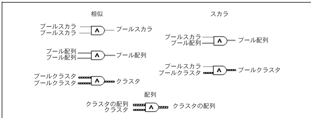
図 B-2 「和」関数のブールの組み合わせ
