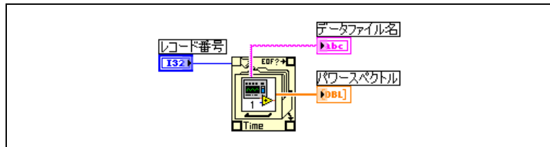
図 14-9 サブ VI の端子を経由したログデータの取り出し
