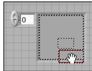
図 10-7 配列シェル
