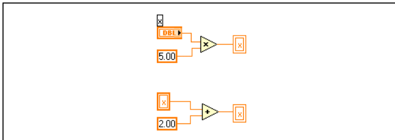
図 11-1 競合状態
