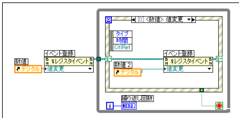
図 9-2 イベント登録を動的に変更する
